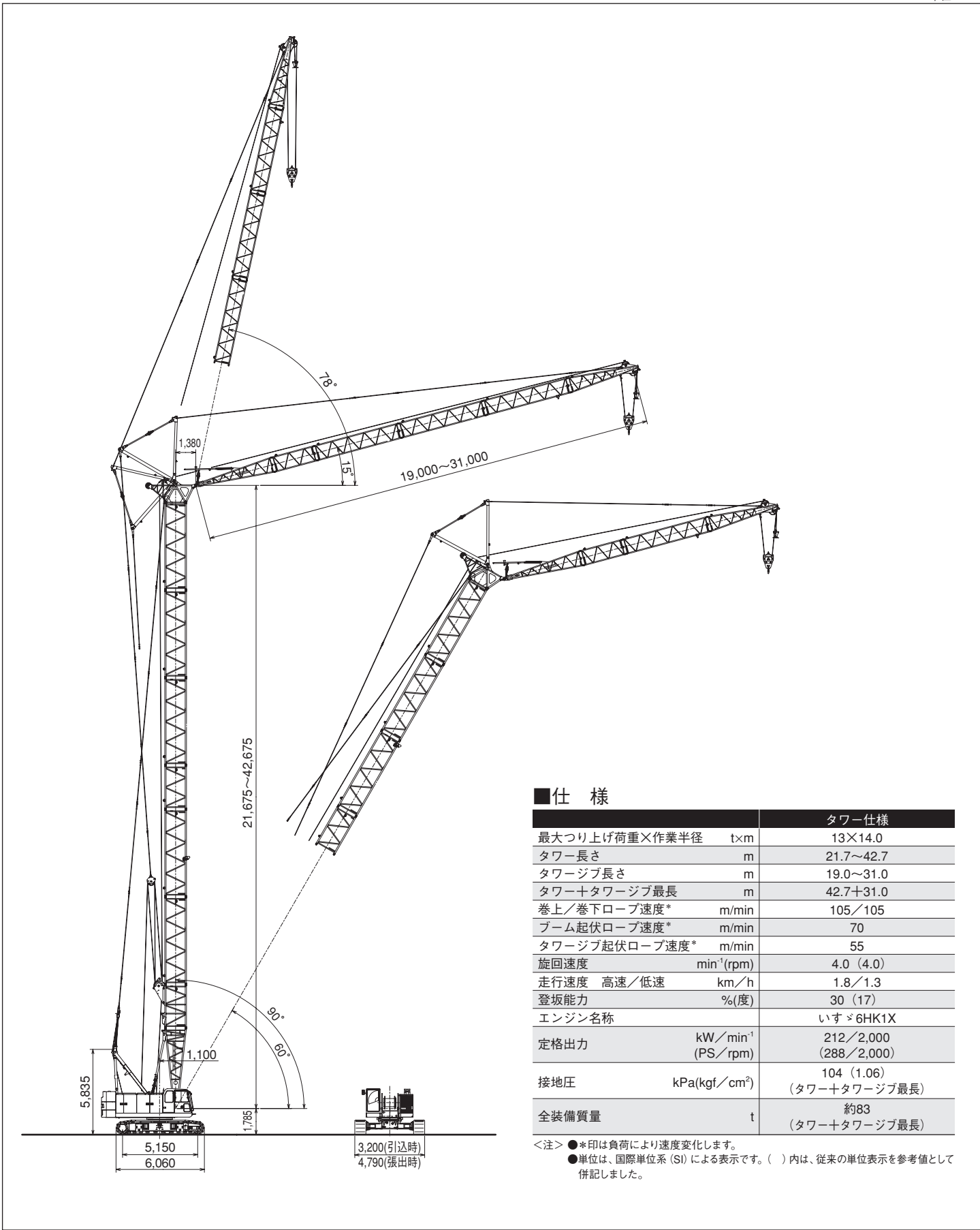
■寸法図
