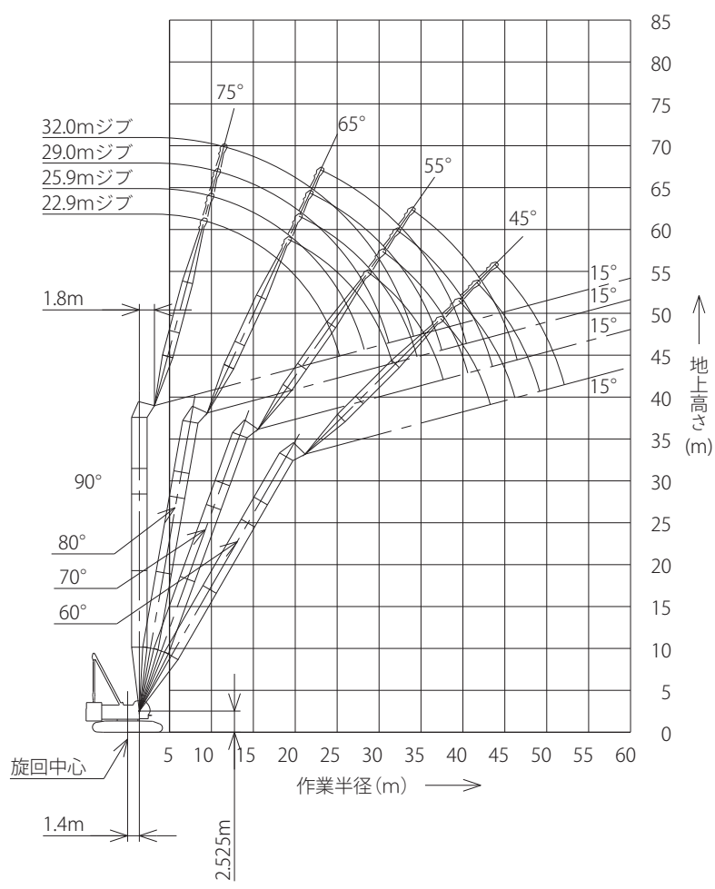
▶ ラッピングタワー定格総荷重表
