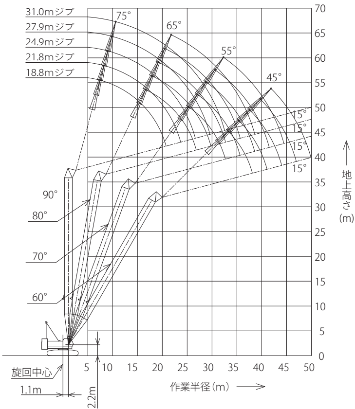
ラッフィングタワー 定格総荷重表 (33.7t カウンタウエイト / カーボディウエイト装着) (単位：t)
